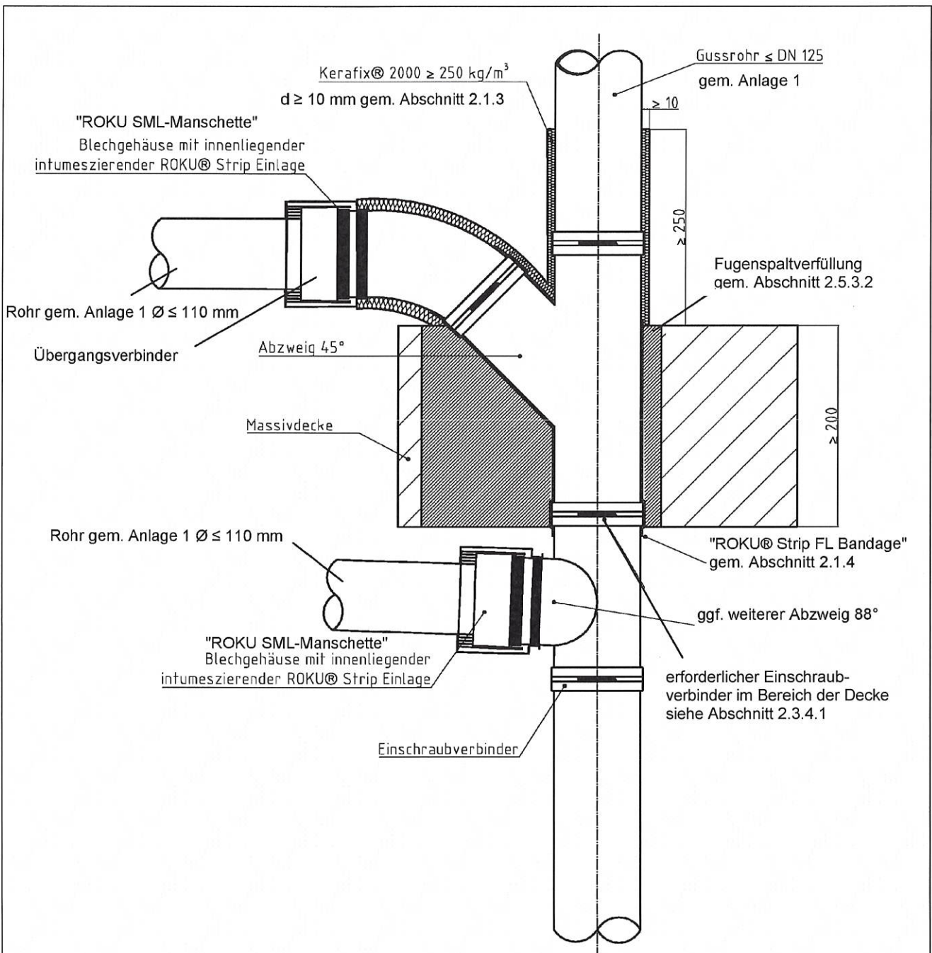
Detail Abzweig s. Anlage 4
