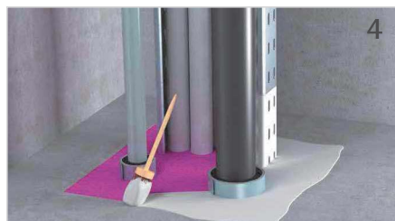
Tangit FP 800 Brandschutz-Anstrich oberhalb des Deckenschotts auf den Schaum und 3 cm des angrenzenden Bereichs, bzw. 15 cm auf die Kabel(-trasse) auftragen.
