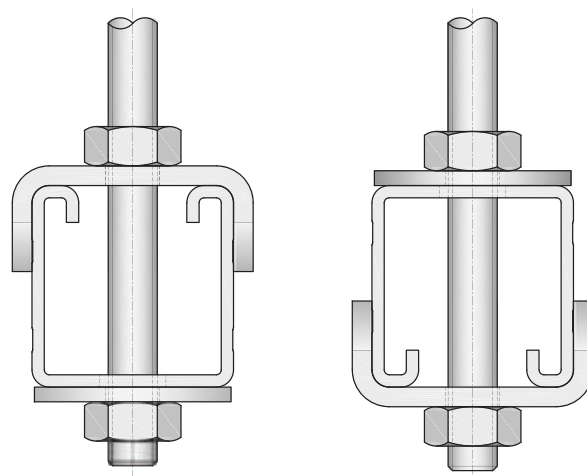
Imagen 3: Uso de la arandela Strut Walraven - en forma de U en el lado abierto del rail
