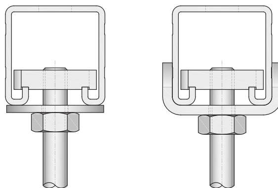
Imagen 4: Aumente la rigidez de las cargas bajo el rail utilizando arandelas en forma de U (imagen derecha) en lugar de arandelas planas estándar (imagen izquierda)
